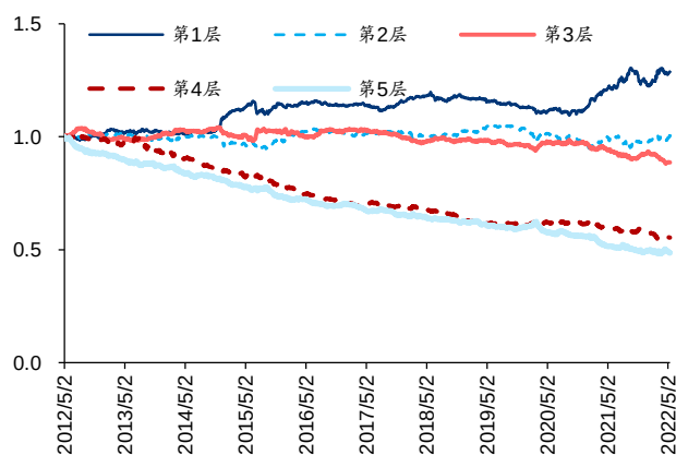
图13: Alpha5 分层测试相对等权基准超额收益(全 A 股内)
