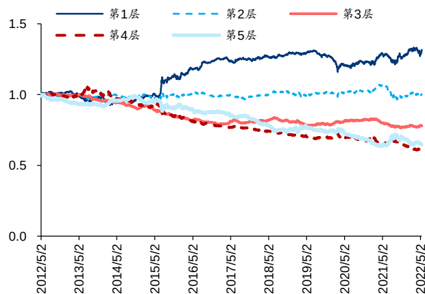
图14: Alpha6 分层测试相对等权基准超额收益(全 A 股内)
