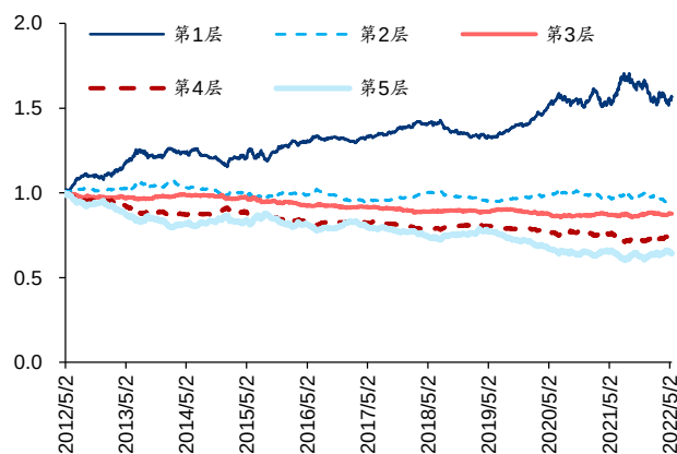
图12: Alpha4 分层测试相对等权基准超额收益(全 A 股内)
