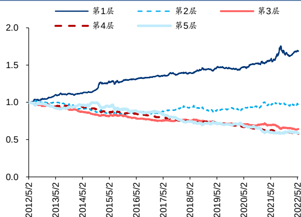
图9: Alpha1 分层测试相对等权基准超额收益(全 A 股内)
