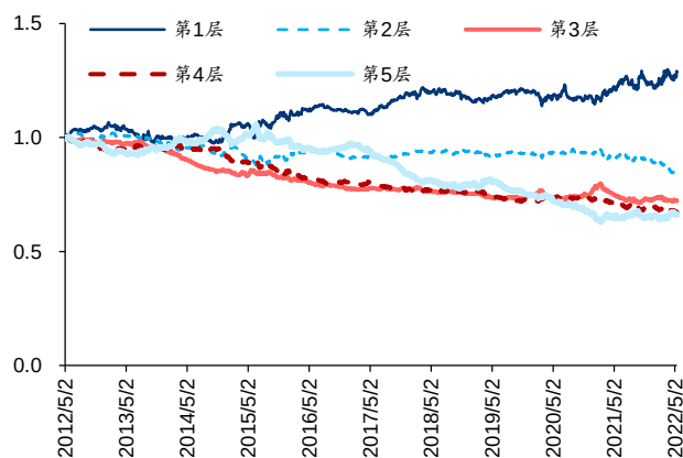
图11: Alpha3 分层测试相对等权基准超额收益(全 A 股内)
