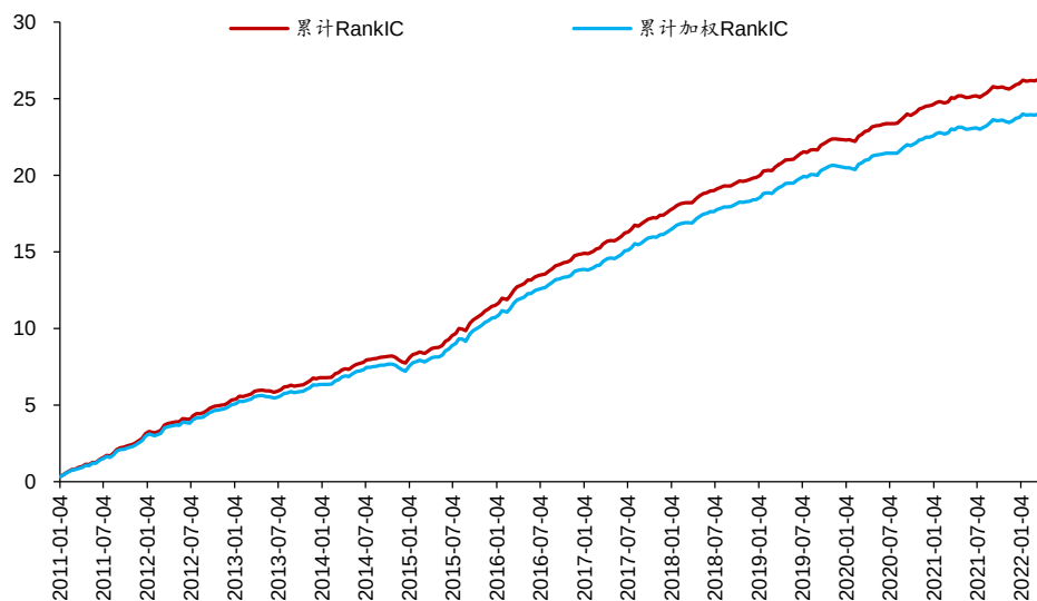
图表4: GAT+residual 模型合成因子累计 RankIC 和加权 RankIC
