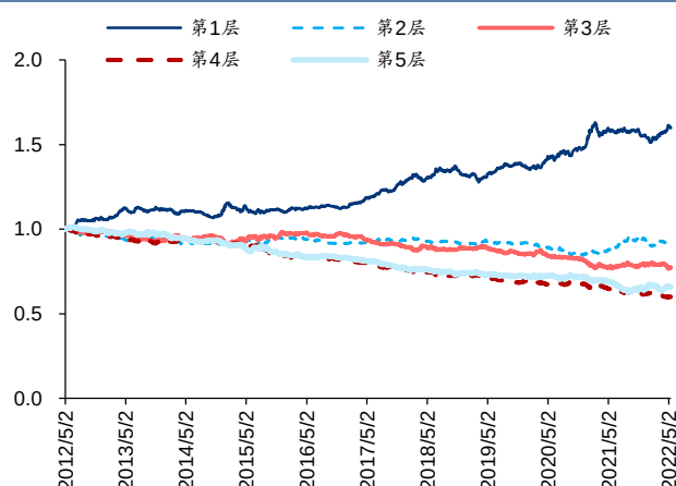
图10: Alpha2 分层测试相对等权基准超额收益(全 A 股内)
