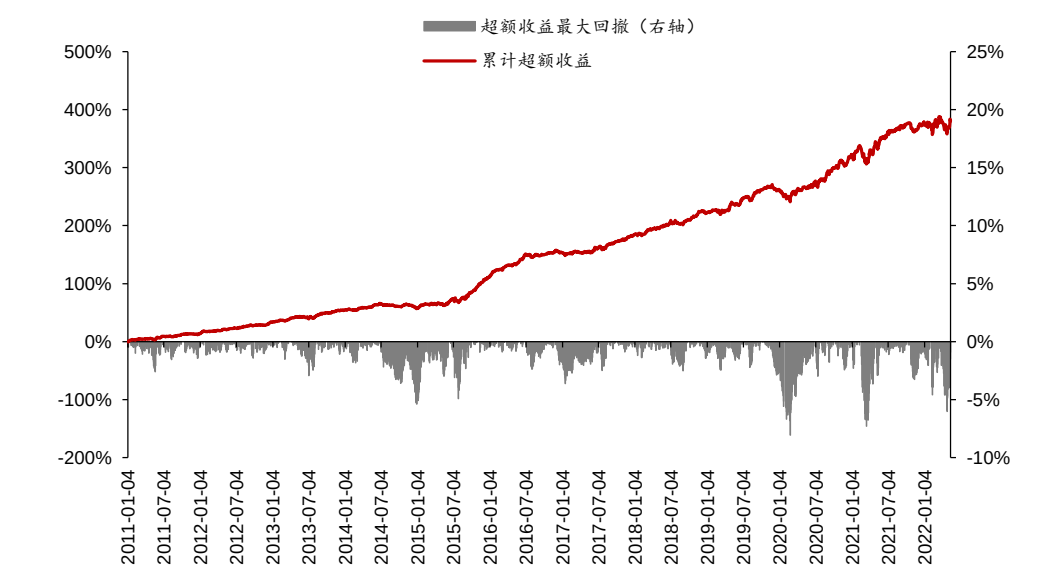
图表1： GAT+residual 模型超额收益表现
